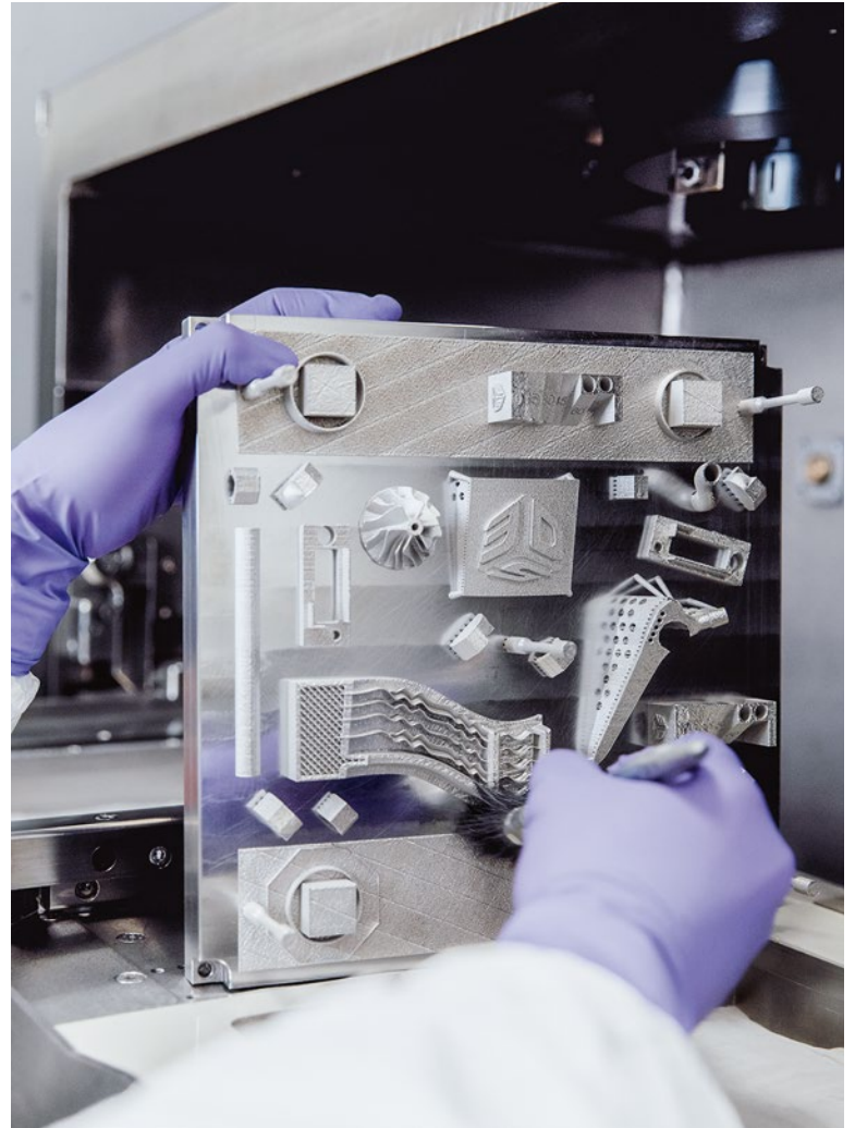
Gedruckte Prüfkörper für die Reaktorentwicklung
